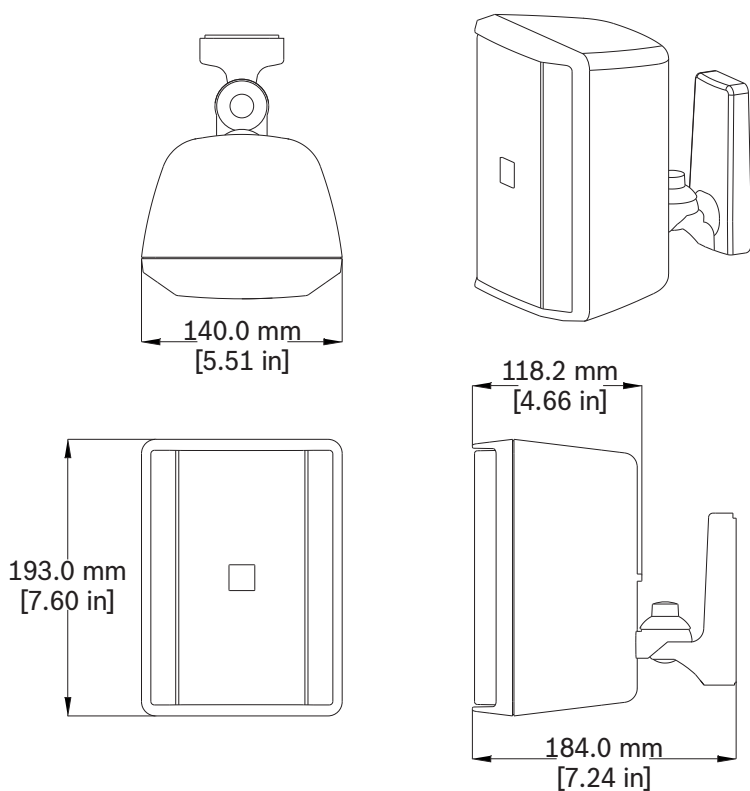
Рис. 6.1: Габариты EVID-S4.2/EVID-S4.2T
