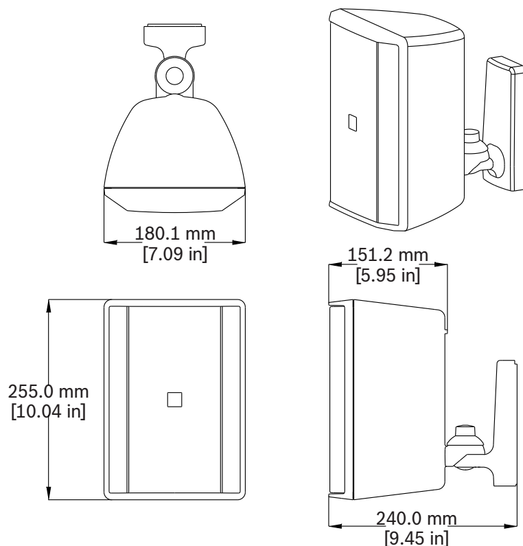
Рис. 6.3: Габариты EVID-S5.2/EVID-S5.2T
