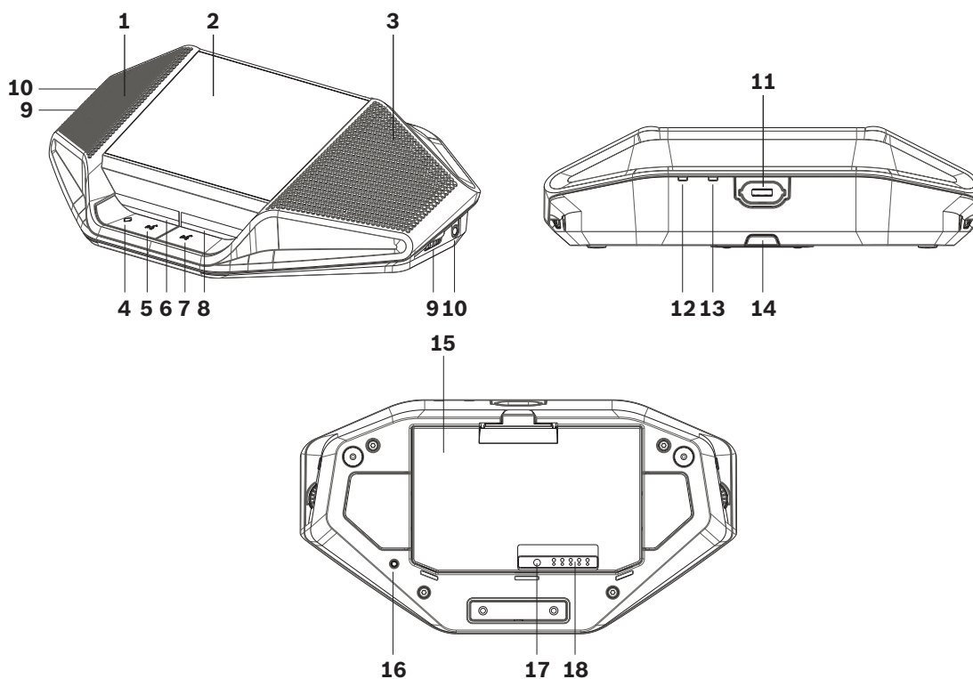
DCNM-WDE и DCNM-WD: вид сверху, сзади и с основания
