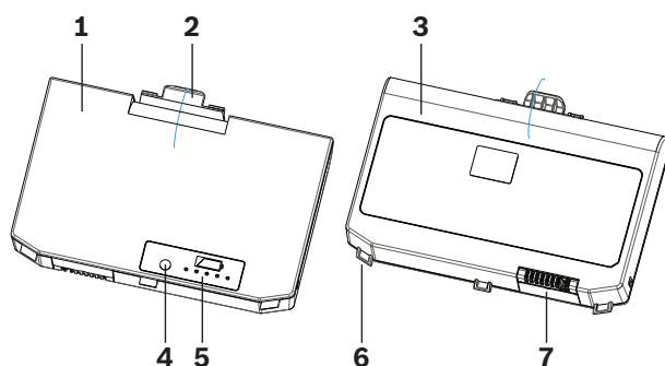
Рис. 6.5: DCNM-WLIION Комплект батарей – вид сверху (1) и сзади (3).
