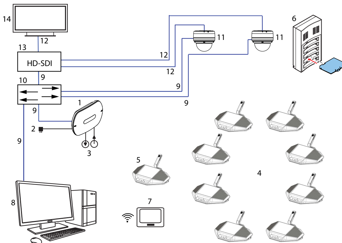
Рис. 3.2: Стандартная Беспроводная конференц-система DICENTIS с расширенными функциональными возможностями
