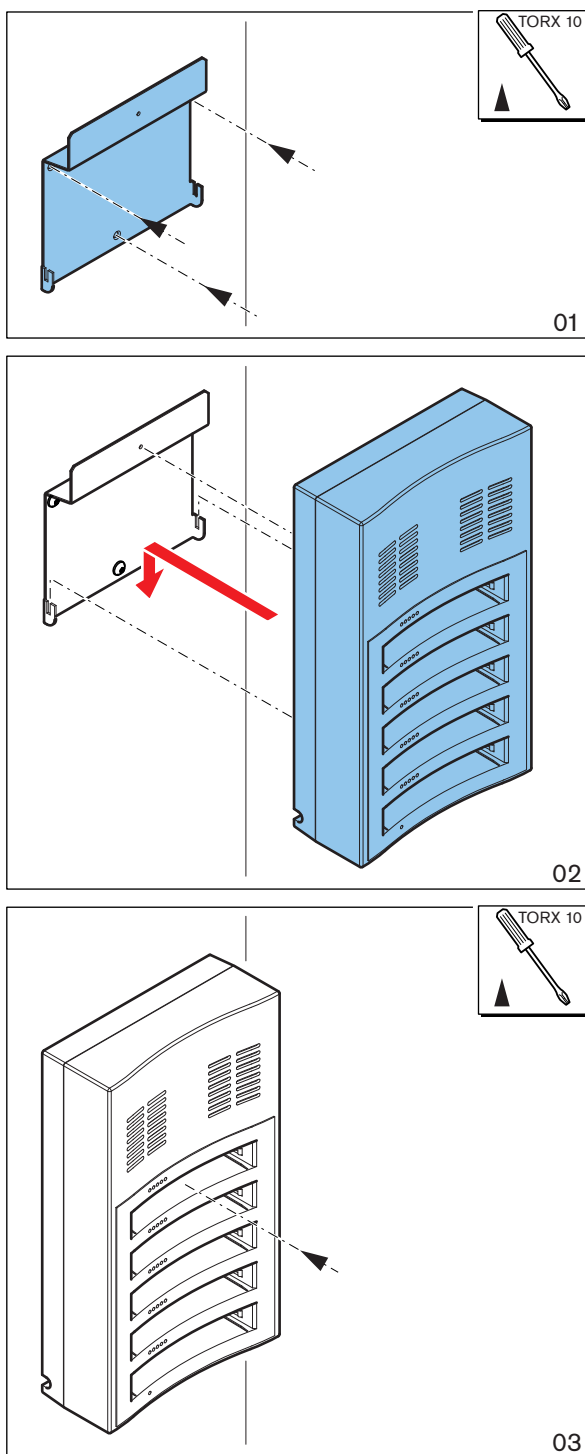
Рис. 6.7: Настенная установка
