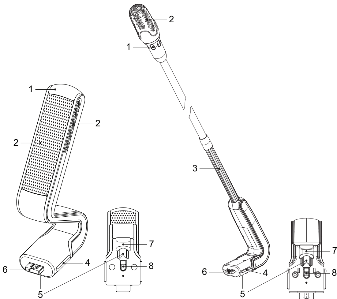
Рис. 6.2: Микрофоны DCNM-HDMIC и DCNM-MICS/DCNM-MICL – вид спереди и снизу
