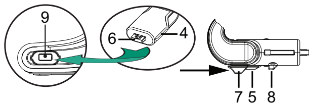
Рис. 6.3: Подключение DCNM-HDMIC или DCNM-MICS / DCNM-MICL
