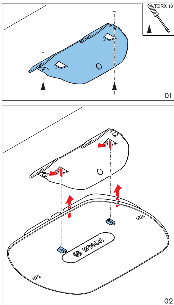
Рис. 5.3: Монтаж на стену или потолок
