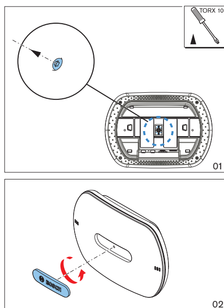
Рис. 5.1: Изменение положение логотипа
