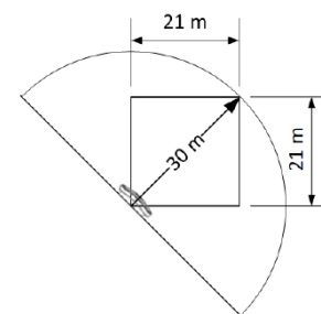
DCNM-WAP Расположение в углу
