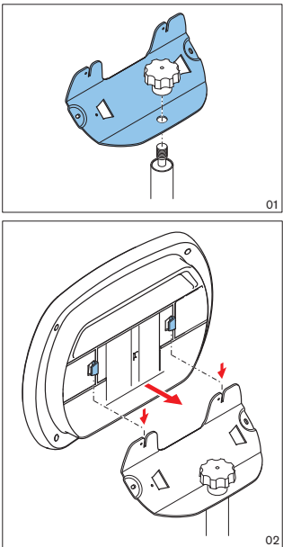
Рис. 5.4: Установка на напольную стойку-треногу
