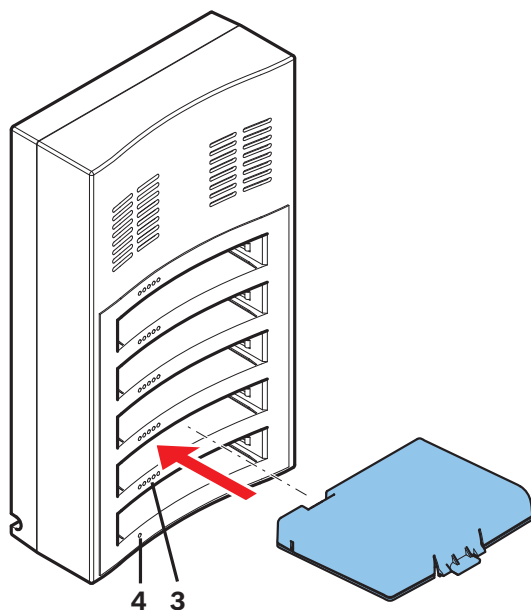
Рис. 6.8: Замена Комплект батарей
