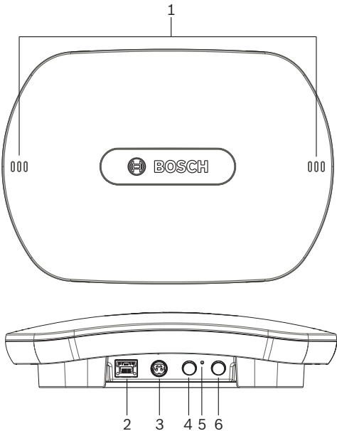
Рис. 5.5: DCNM-WAP – вид спереди и снизу
