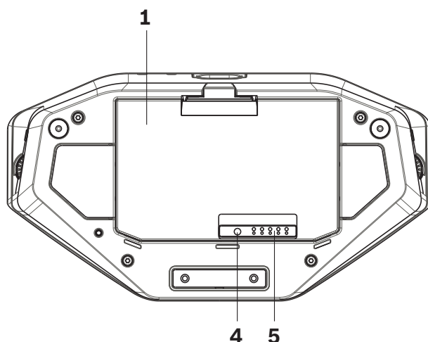
Рис. 6.4: Беспроводное устройство – вид снизу, включая Комплект батарей
