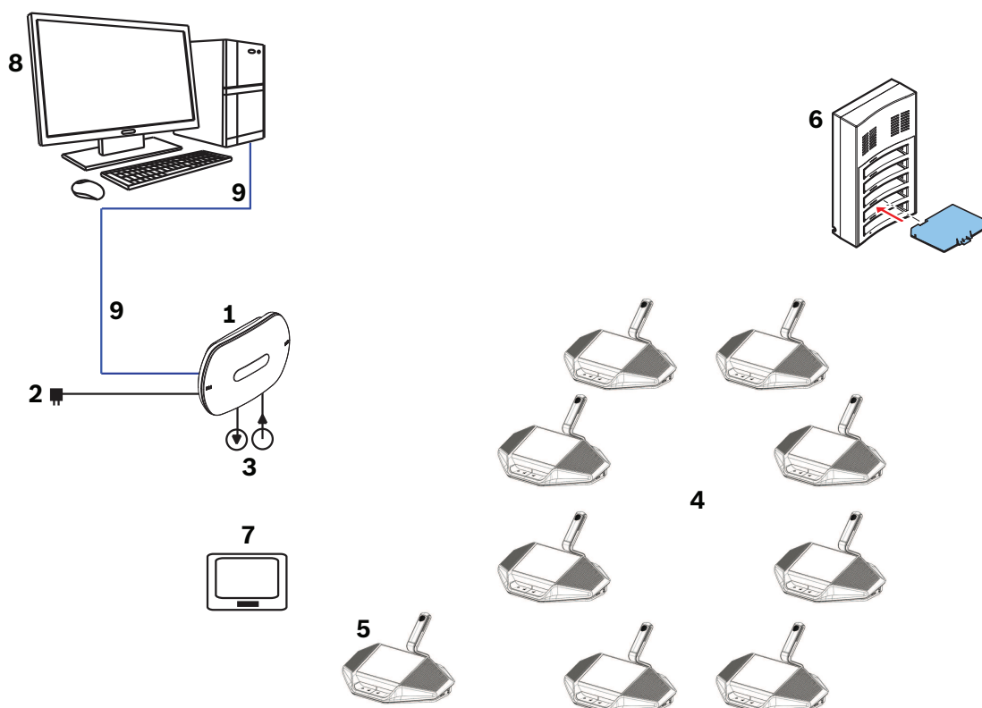
Рис. 3.1: Стандартная Беспроводная конференц-система DICENTIS
