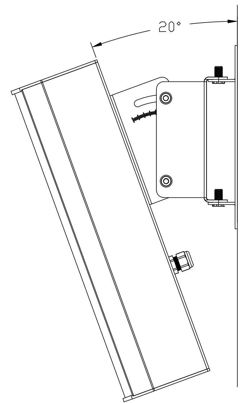
UBX4 TILT RANGE
